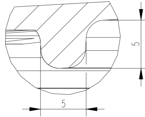
DETAIL A SCALE 4:1 TYP 3 PLCS
